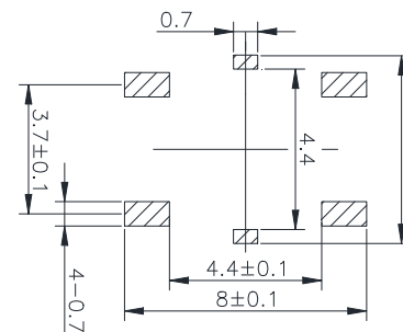
PCB. 焊接图
