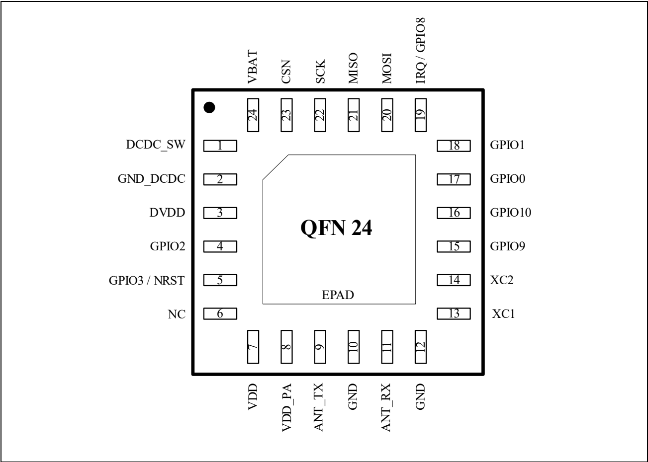
图 4-1 QFN24 引脚图
