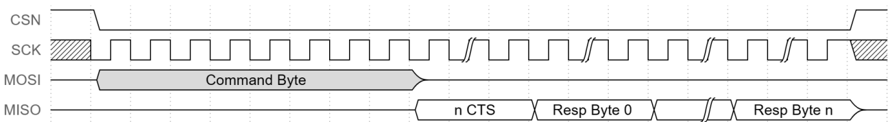
图 7-4 读命令时序
