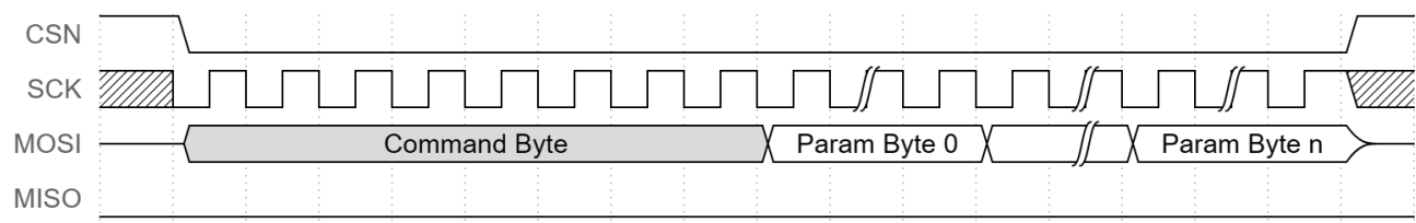
图 7-3 写命令时序
