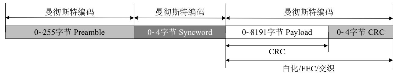
图 9-2 固定包长帧结构
