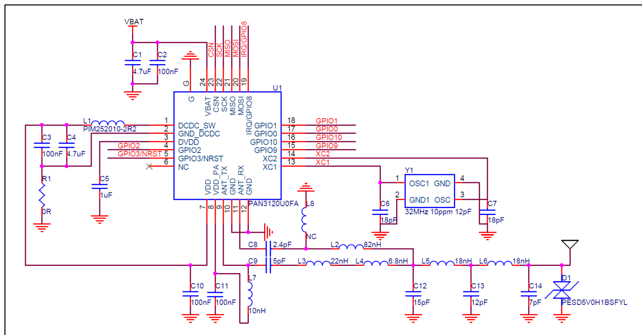
图 11-1 参考原理图
