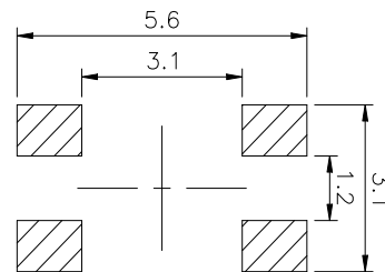
PCB. 焊接图
