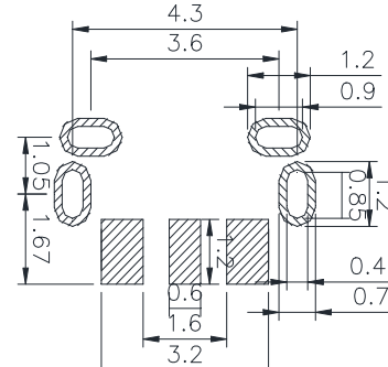
PCB. 焊接图
