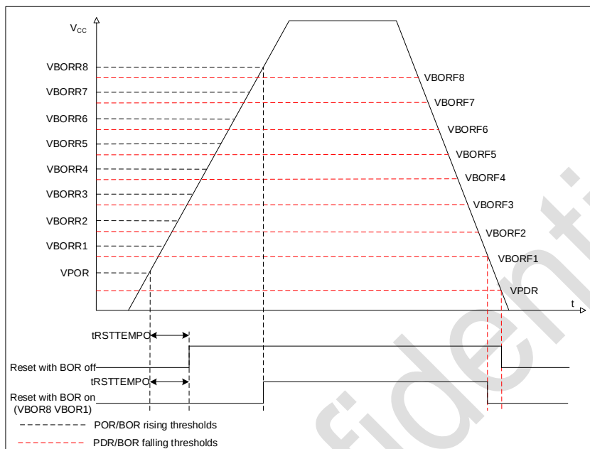
图 2-3 POR/PDR/BOR 阈值
