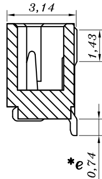
截面 A-A
