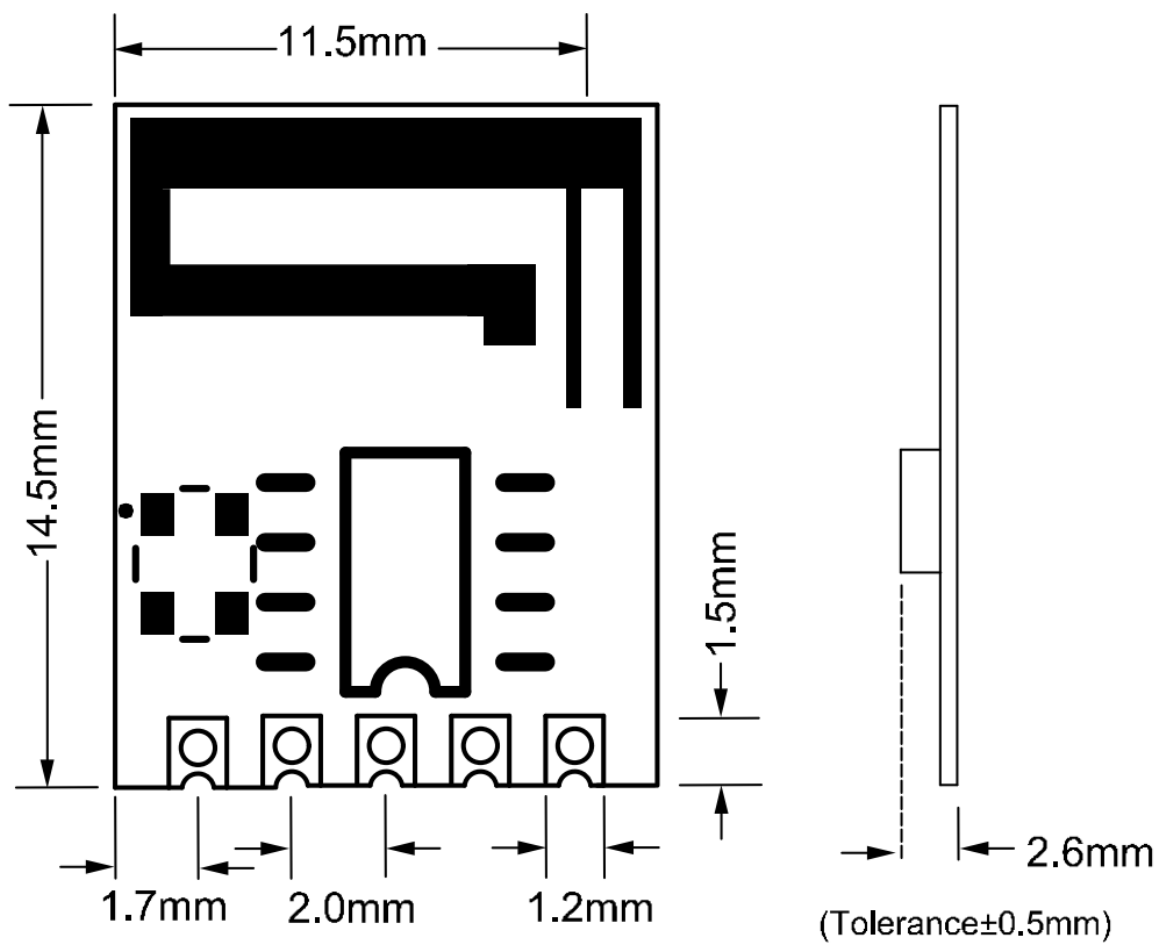
图 3-1：模组尺寸
