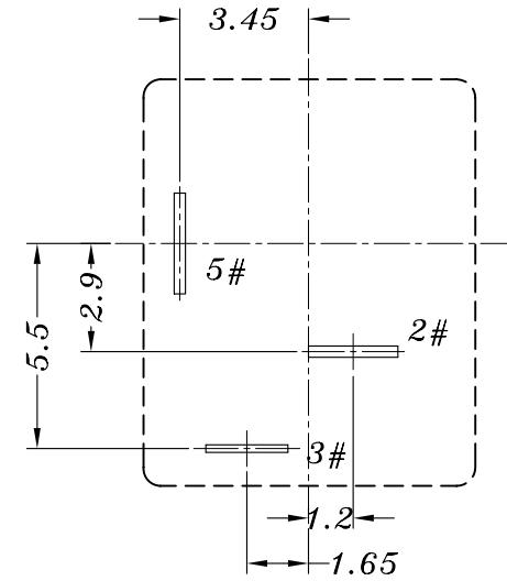
P.C.B LAYOUT
