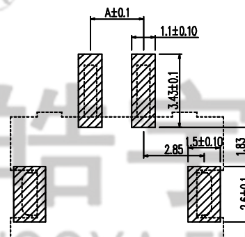
印制线路板
