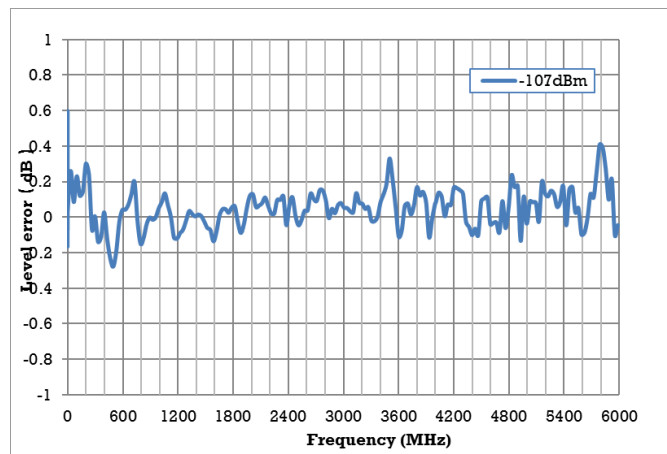
电平误差 VS 频率，输出电平= -107 dBm
