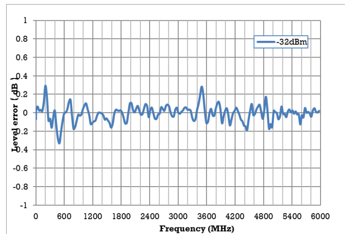
电平误差 VS 频率，输出电平= -32 dBm
