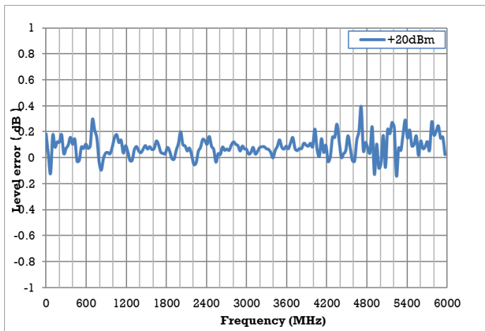
电平误差 VS 频率，输出电平= 20 dBm
