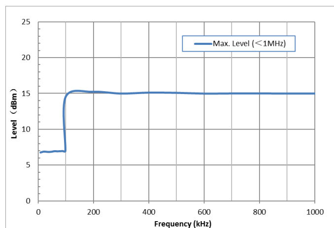
最大输出功率 VS 频率, f < 1 MHz
