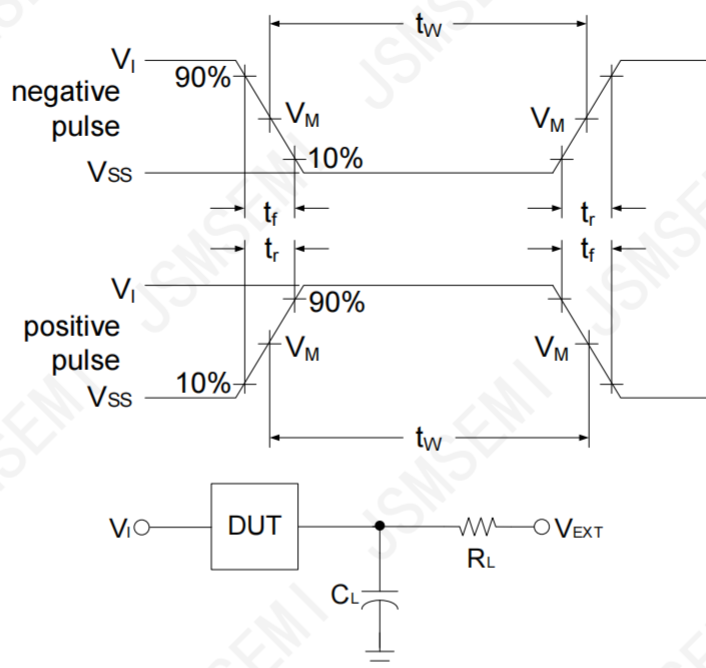
图2 负载线路
