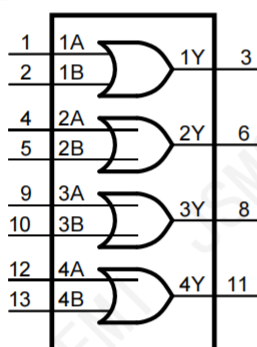
图 1 逻辑符号
