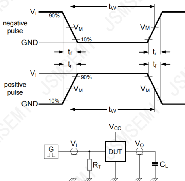
图4 测量开关时间的测试电路
