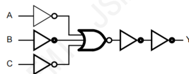
图 3 逻辑框图（单路）
