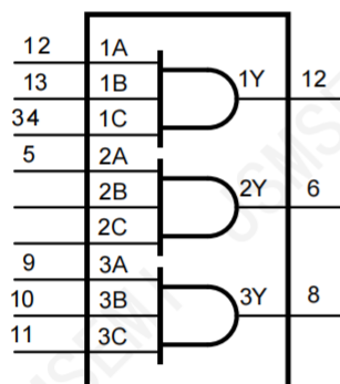
图 1 逻辑符号
