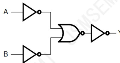
图 3 逻辑框图
