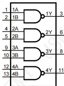
图 1 逻辑符号
