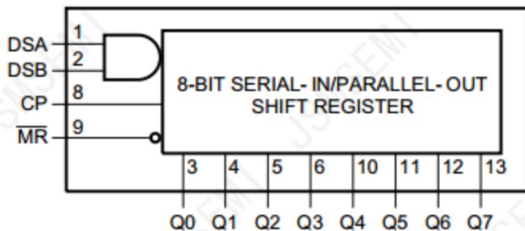
图 3 逻辑框图
