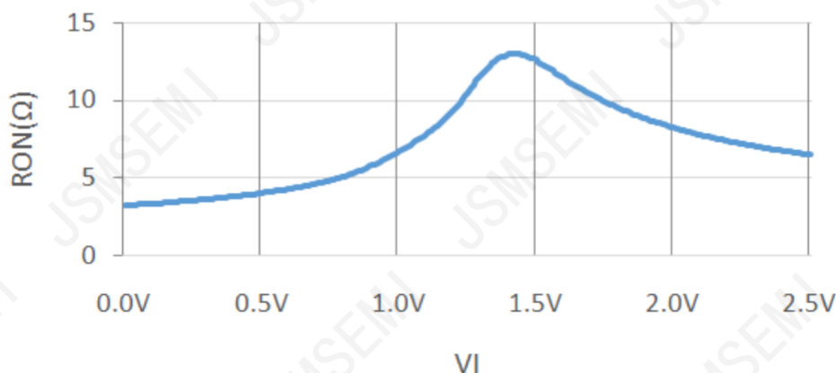
图3 导通电阻与输入电压的关系 ( V_{CC}=2.5\text{V} , I_{sw}=24\text{mA} , T_{amb}=25^{\circ}\text{C} )
