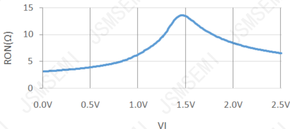
图2 导通电阻与输入电压的关系 ( V_{CC}=2.5\text{V} , I_{sw}=15\text{mA} , T_{amb}=25^{\circ}\text{C} )
