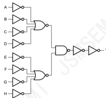
图3 逻辑框图
