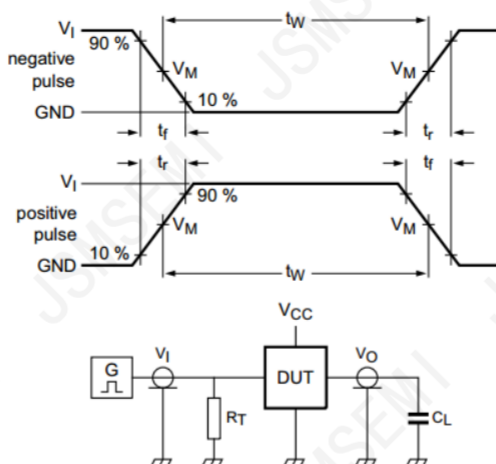
图 4 测试开关时间电路
