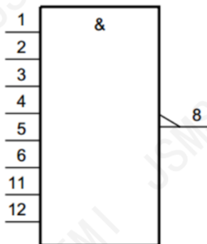
图2 IEC 逻辑符号
