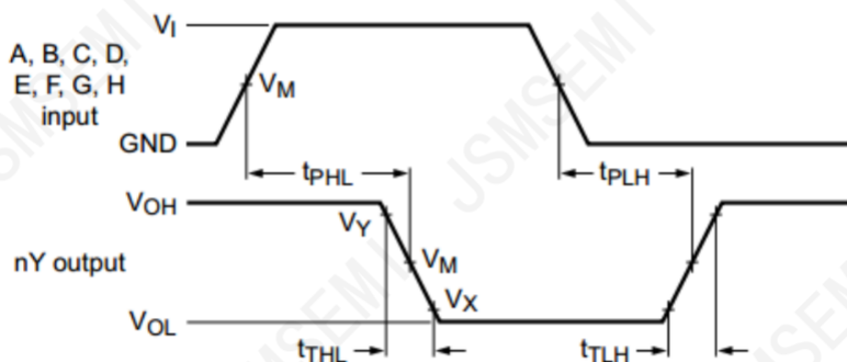
图 5 输入到输出传输延时和输出转换时间
