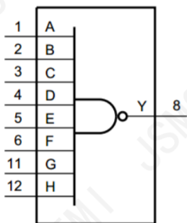
图1 逻辑符号
