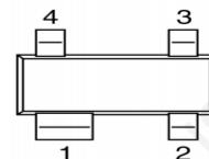
SOT143
