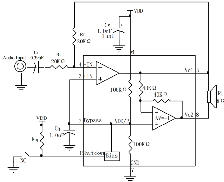
图 1、HX4871 典型应用图
