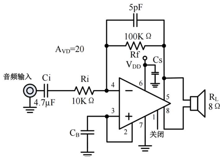
图 2、高增益电路
