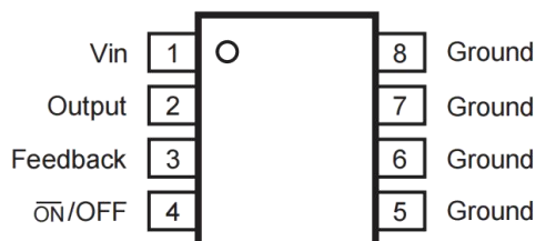
LM2575M-XX
