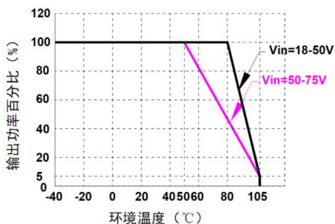
温度降额曲线图 (HVQ40-48S12/24V3) 图 2-2
