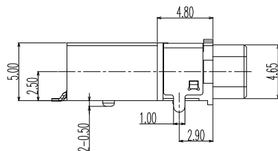
面板开孔参考尺寸
