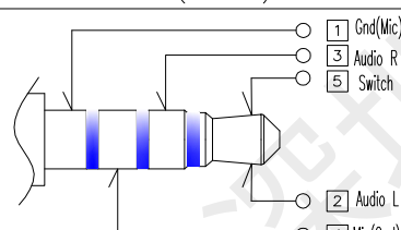
SCHEMATIC(PLUG IN)
