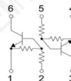
SOT-363
