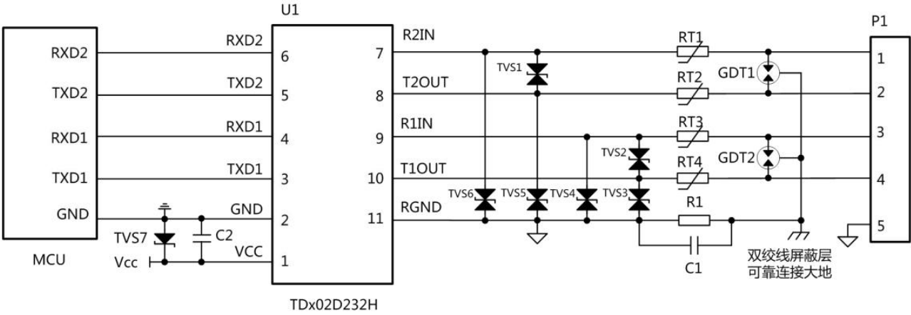
图 2. EMC 推荐电路
