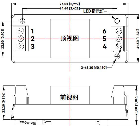
HVQ10-xxSxxV3CR 尺寸图
