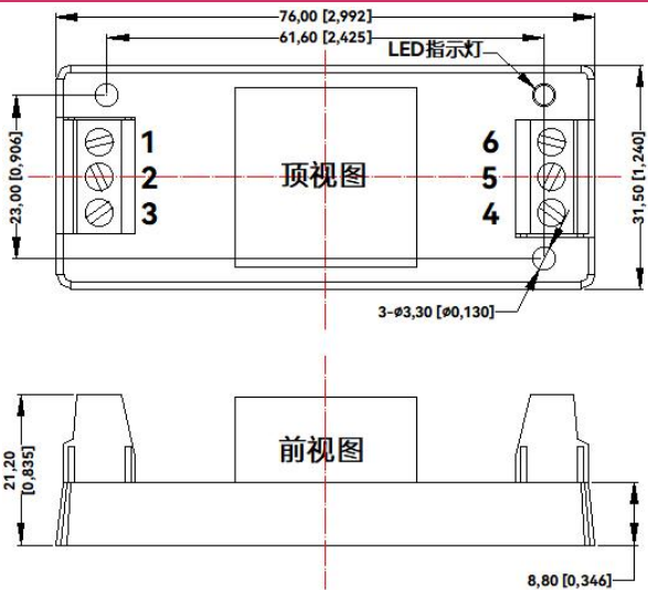
HVQ10-xxSxxV3CW 尺寸图
