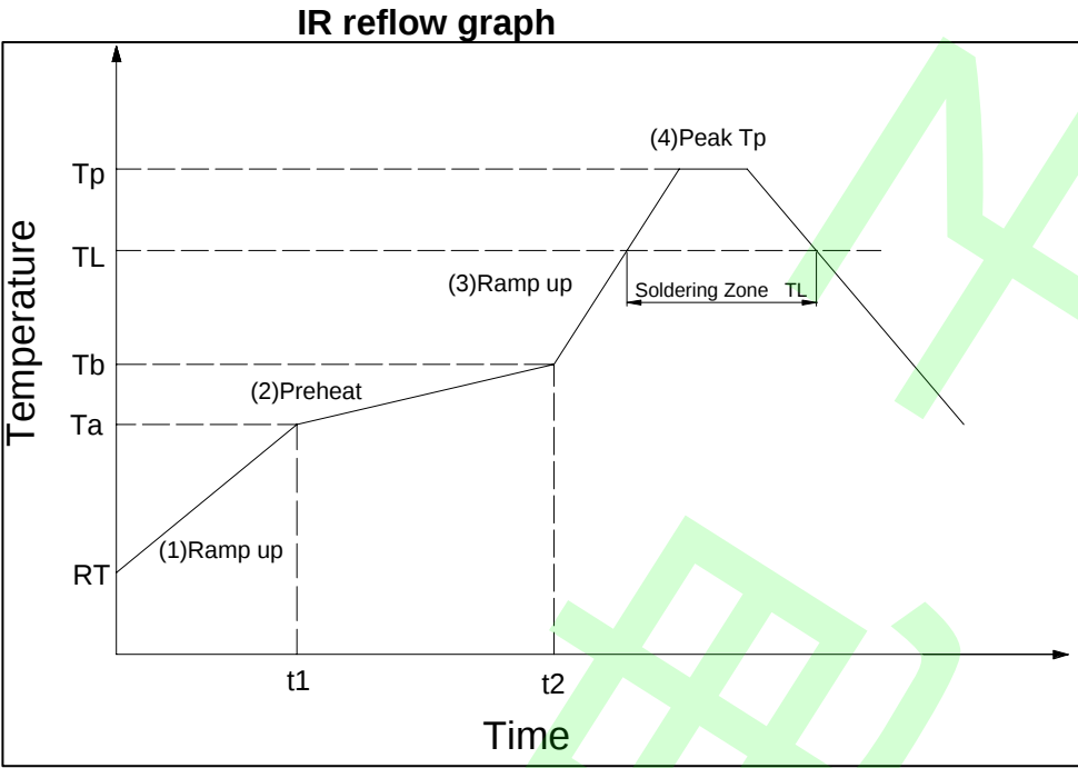
IR reflow profile
