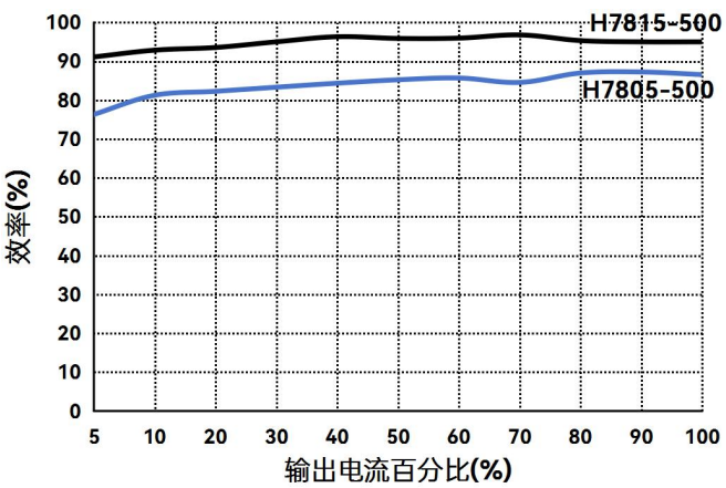
负输出效率 VS 输出负载曲线图 (标称输入)
