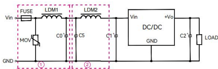
EMC 推荐电路（图 5）
