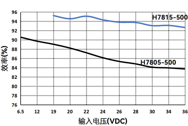
负输出效率 VS 输入电压曲线图 (满载)
