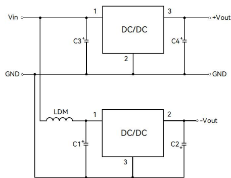
EMC 推荐电路（图 5）
