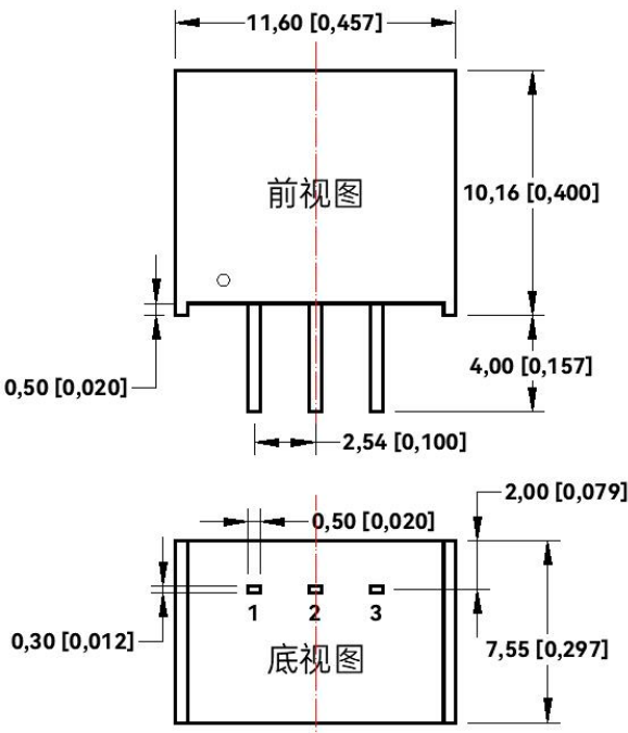
外观尺寸图
