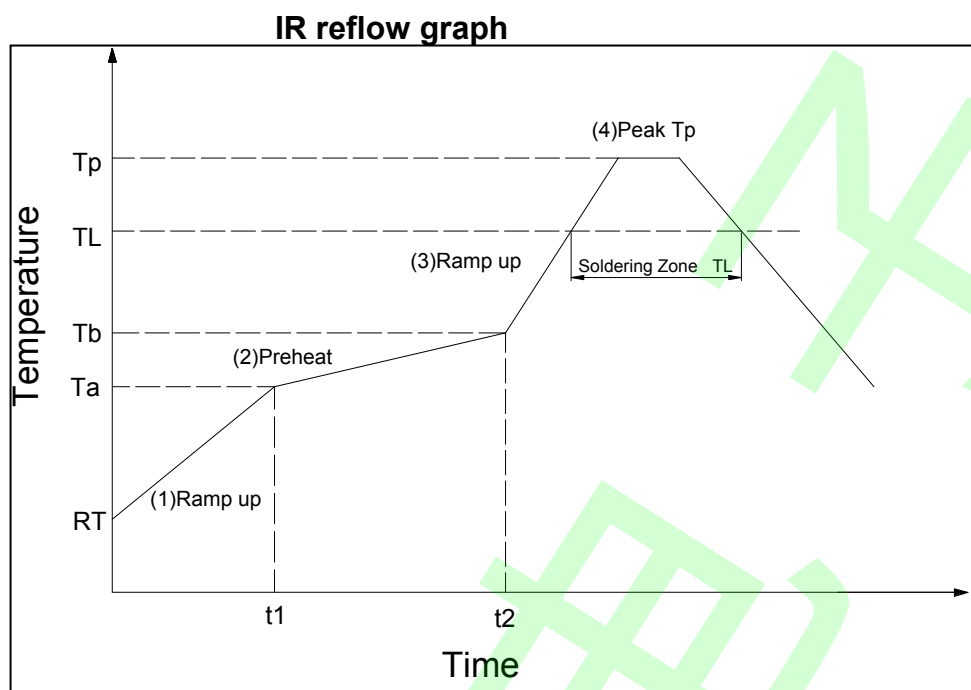
Form-1 (Reference JEDEC J-STD-020C Table 5-2) )
