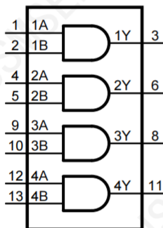
图 1 逻辑符号
