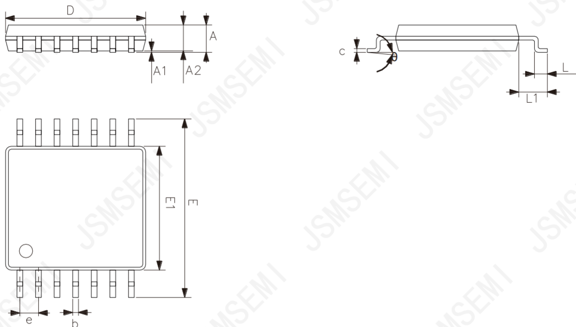
TSSOP14 外形图与封装尺寸
