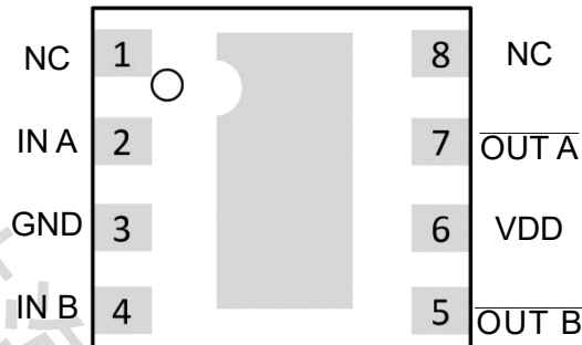
SOP8
