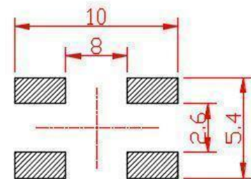
PCB. 焊接图
