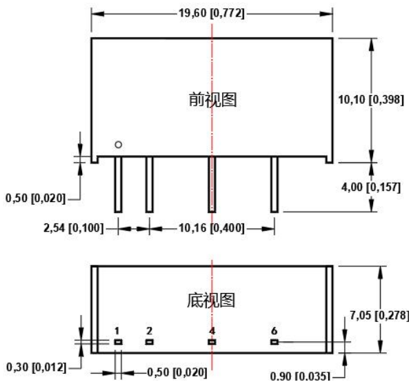
外观尺寸图
