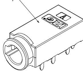
不带防水圈
