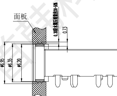
面板开孔建议尺寸 (Ø6.35)
