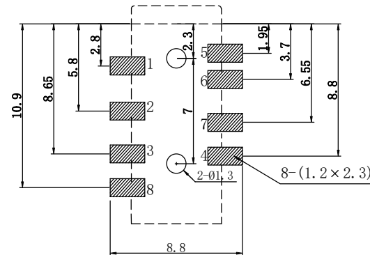
电路板开孔尺寸
