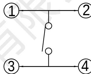
原理图
