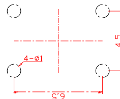
PCB. 焊接图
