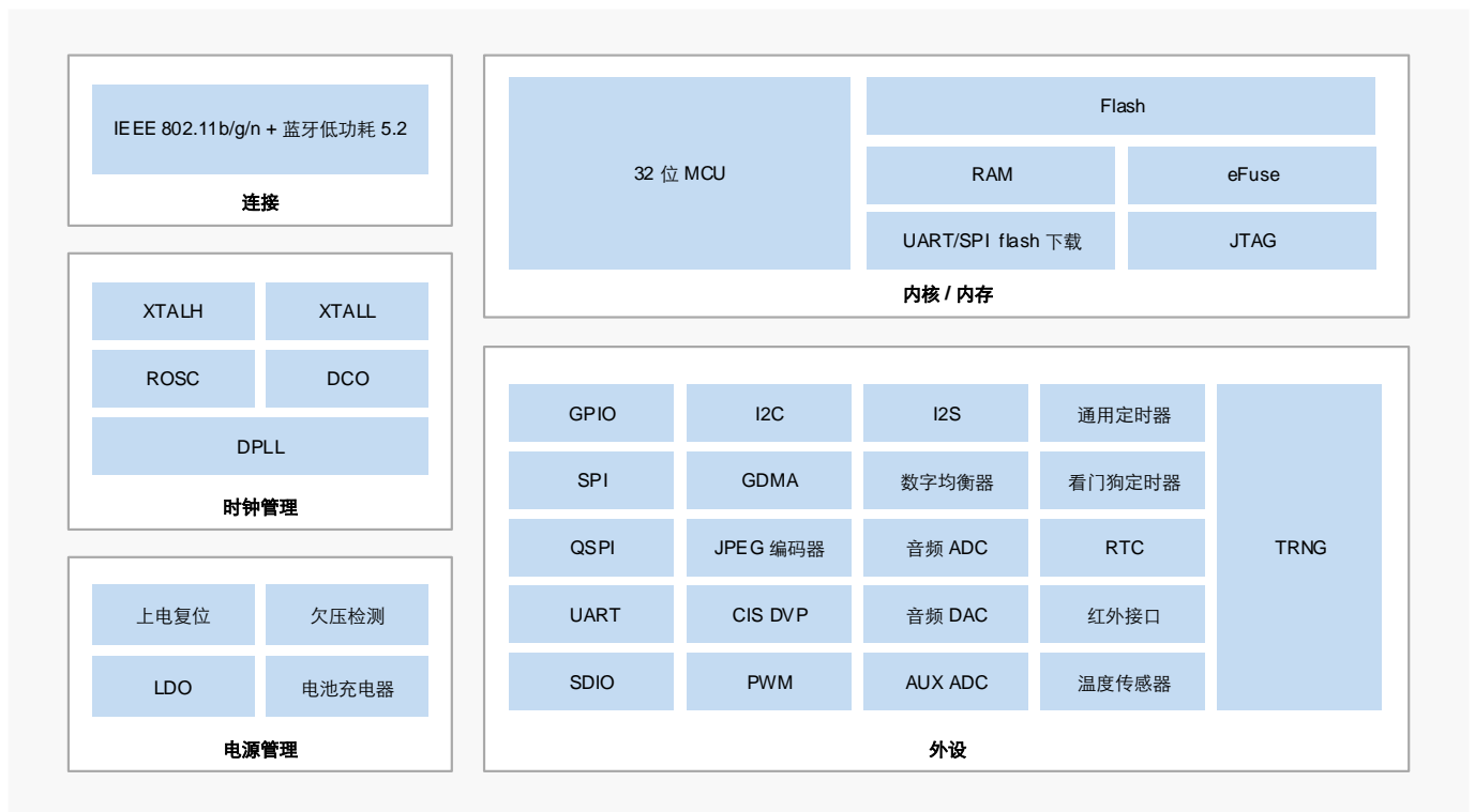
图 2-1 BK7252N 框图
