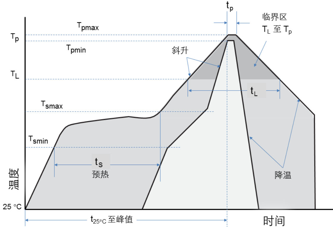
图 7-1 回流焊曲线
