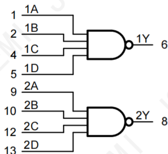
图 1 逻辑符号
