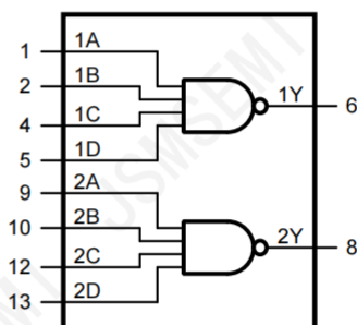
图 4 功能框图
