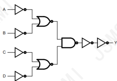
图 3 逻辑框图
