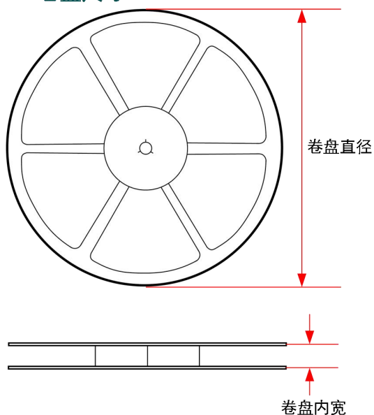
卷盘尺寸
