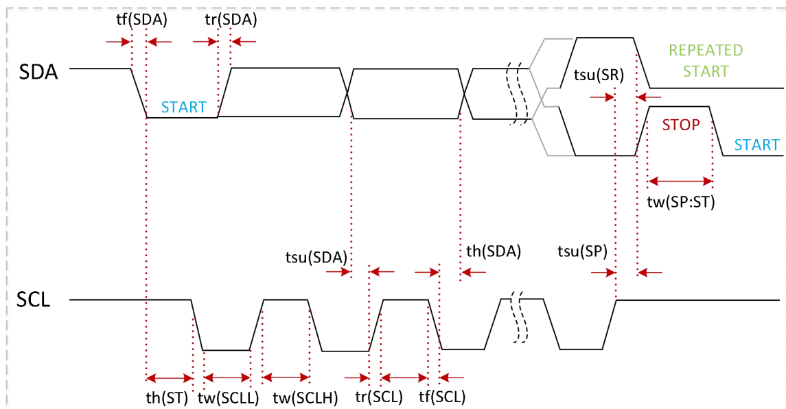
图 13-1 I2C 时序图
