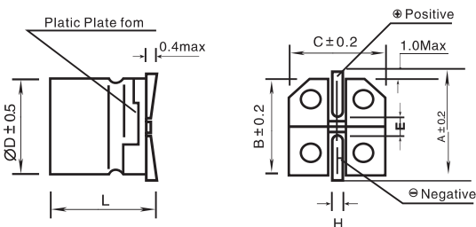
Fig. 2 (≥Φ16.5)
