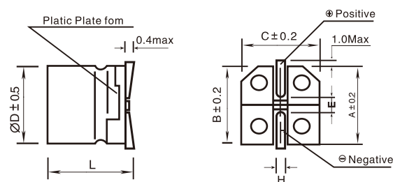
Fig. 2 (≥Φ12.5)
