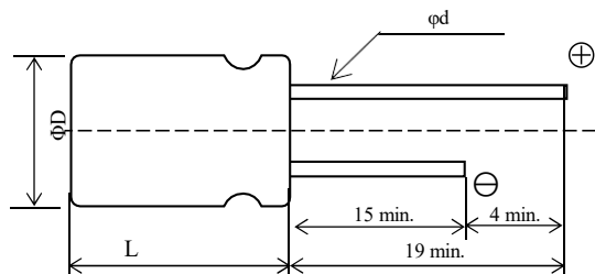
◆尺寸图 [mm]
