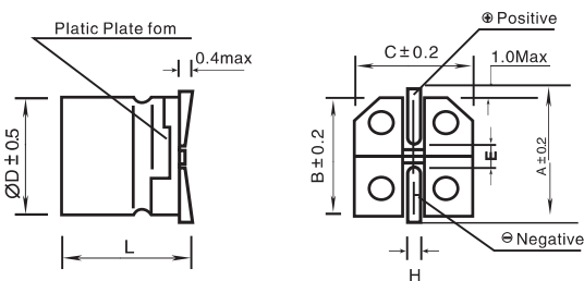
Fig. 2 (≥ Φ16.5)
