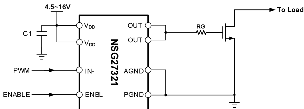
图 9-2 NSG27321 典型应用电路图
