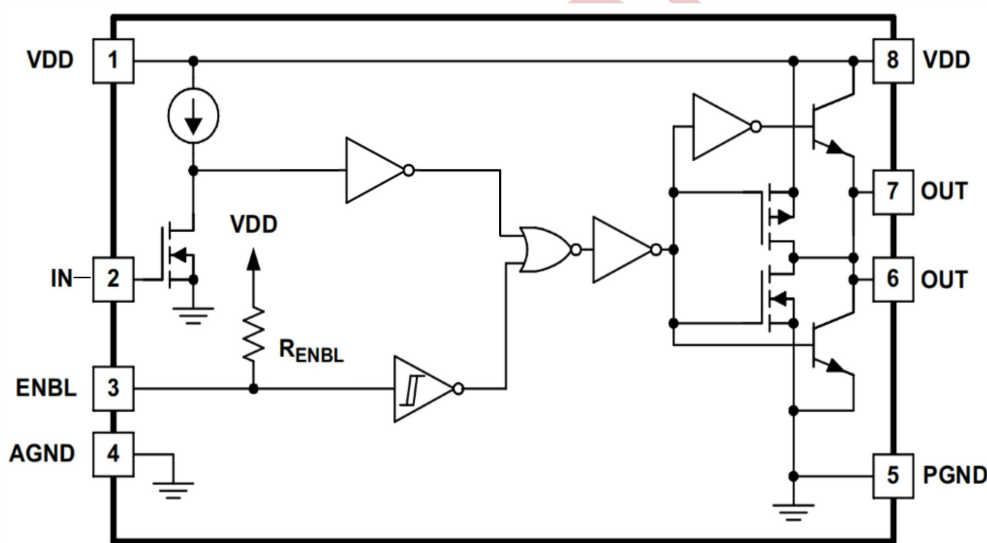
图 9-1 NSG27321 功能框图
