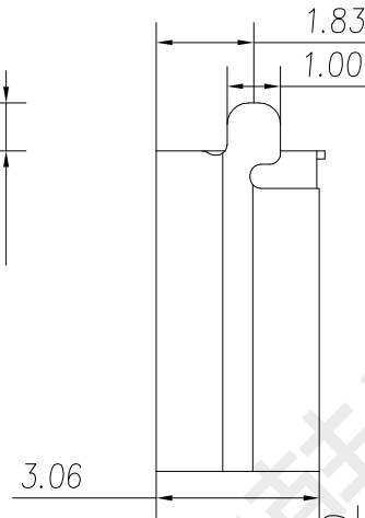
剖面: A-A
