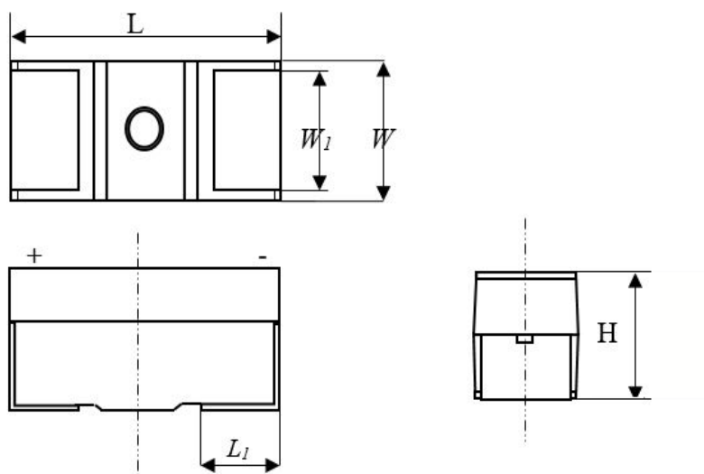
图1 电容器的外形示意图
