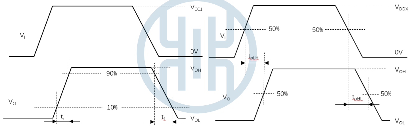
图 13. 传输时间波形测量
