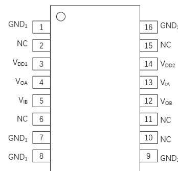
图 8. \pi 122\text{U}6\text{x} 管脚定义
