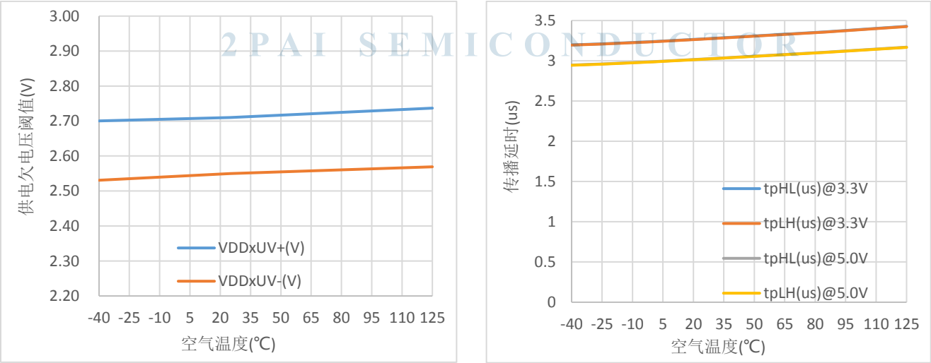
图 10.UVLO vs. 空气温度
