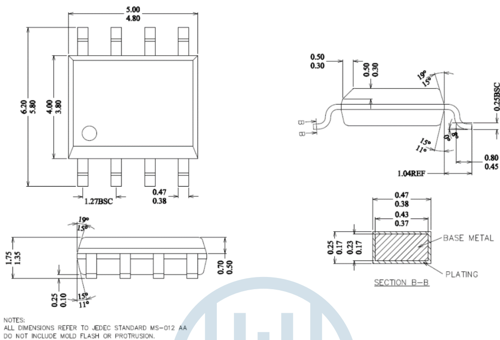
图 17. NB SOIC-8 封装外形尺寸-尺寸单位(mm)
