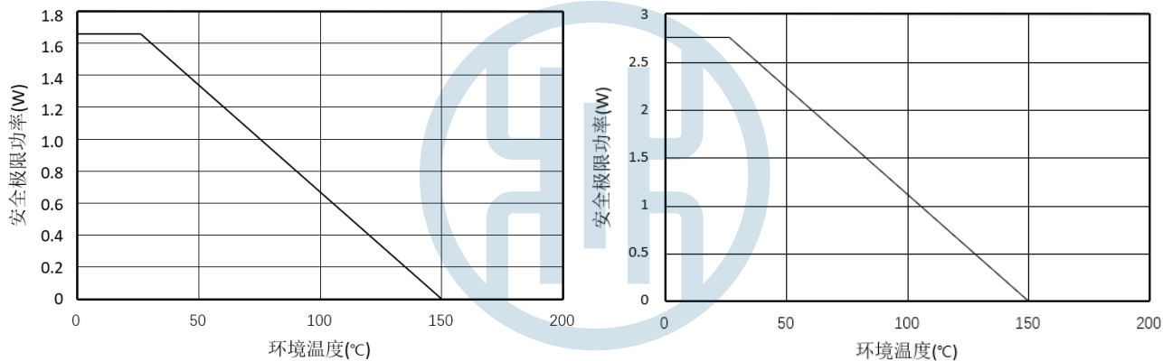
图 9.热降额曲线，依据 DIN V VDE V 0884-11 的安全限值与环境温度的关系(左: π12xU3x; 右: π12xU6x)
