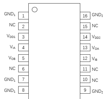
图 7. \pi 121\text{U}6\text{x} 管脚定义
