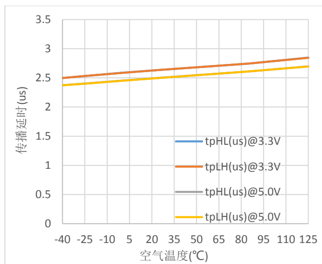
图 12. \pi 12xU6x 传输延时 vs. 空气温度
