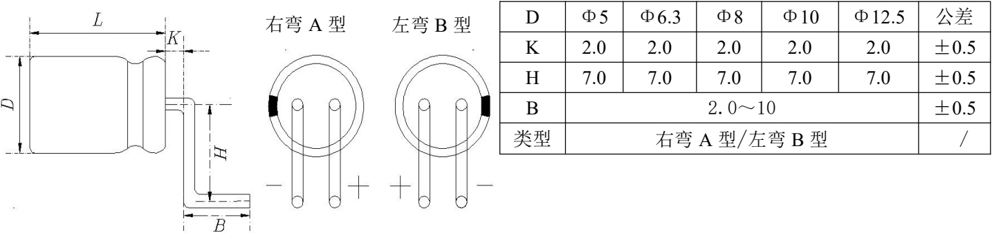
脚成型 H 图（成型双折弯 90°）
