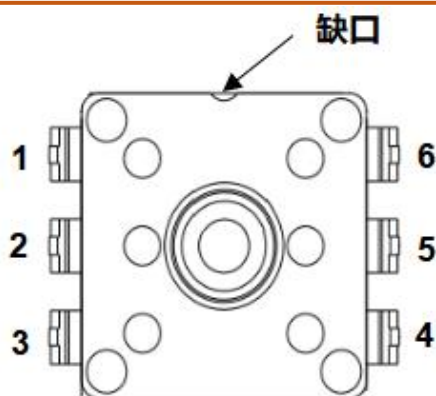
图 7：引脚定义图
