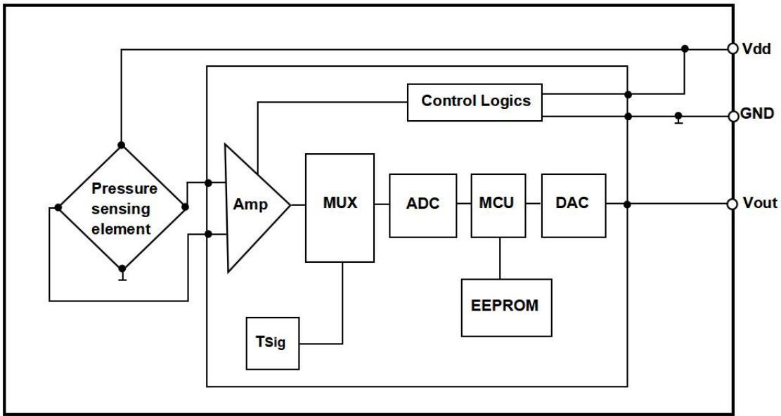
图 1: HBP1201A-4 产品框图
