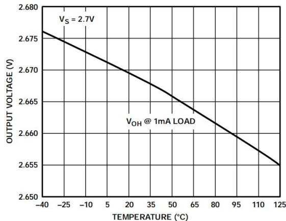
图35. 输出电压高摆幅与温度的关系
