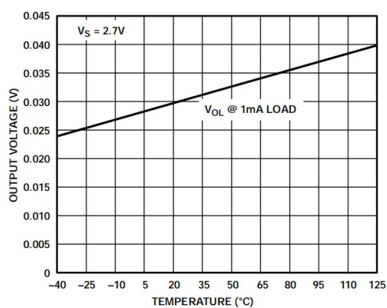
图36. 输出电压低摆幅与温度的关系
