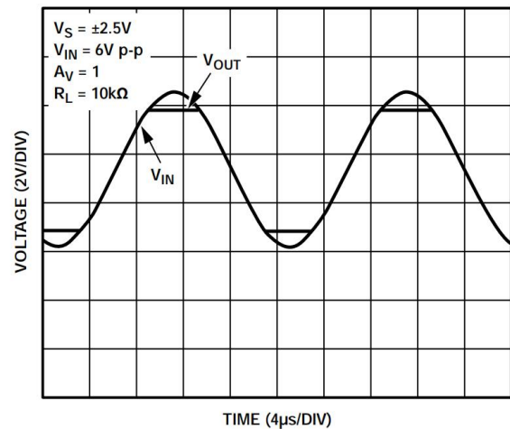
图44. 无反相
