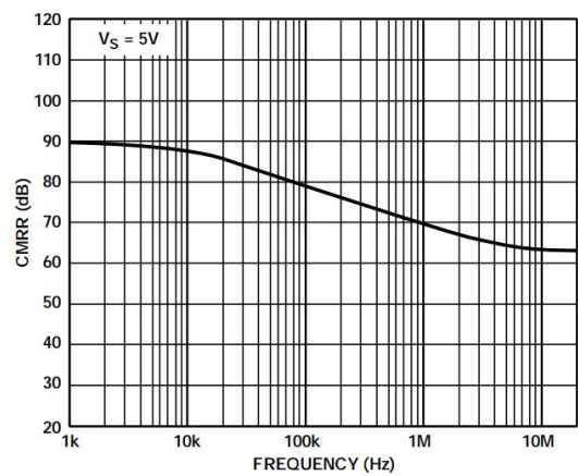
图18. 共模抑制比(CMRR)与频率的关系
