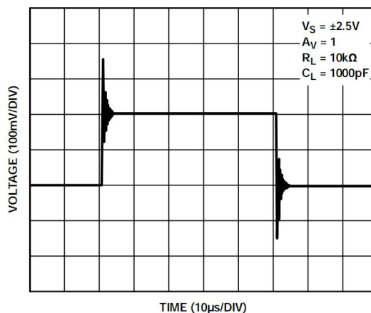
图48.HGV752 无缓冲器情况下的容性负载驱动
