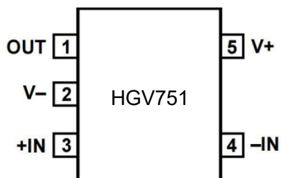
图 1. SOT-23-5 (M5 后缀)
