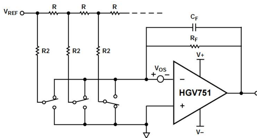
图 56. DAC8143 利用 作为输出缓冲器的电路示意图
