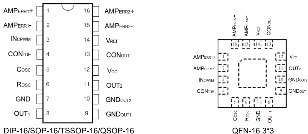
图 2 TL494A 管脚 (顶部视图)
