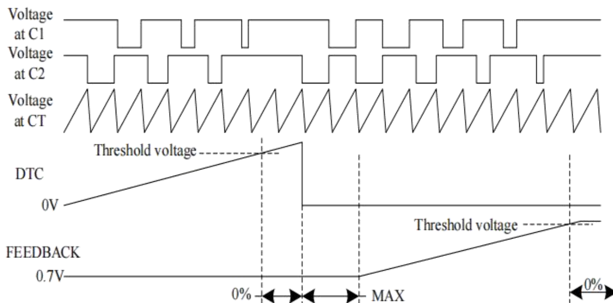
图 6 电压波形
