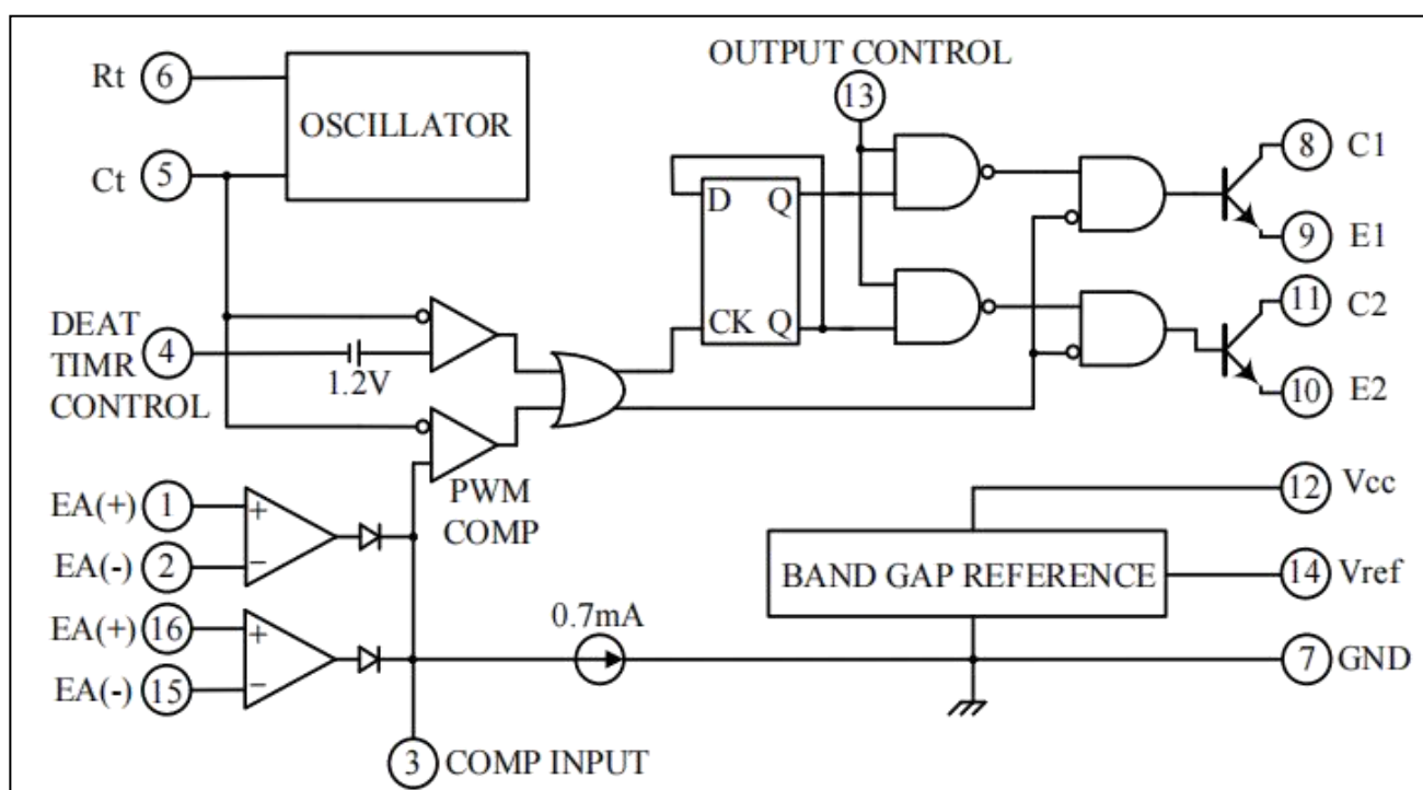
图 1 TL494A 原理图
